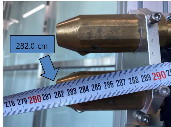
그림 13) 시험품 장착 사진 (거리 측정, 확대)
