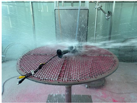
그림 16) 시험 진행 사진
