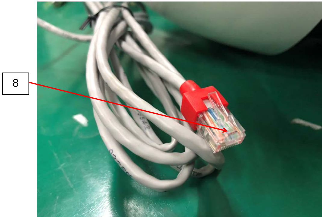
[시험기자재 포트]
