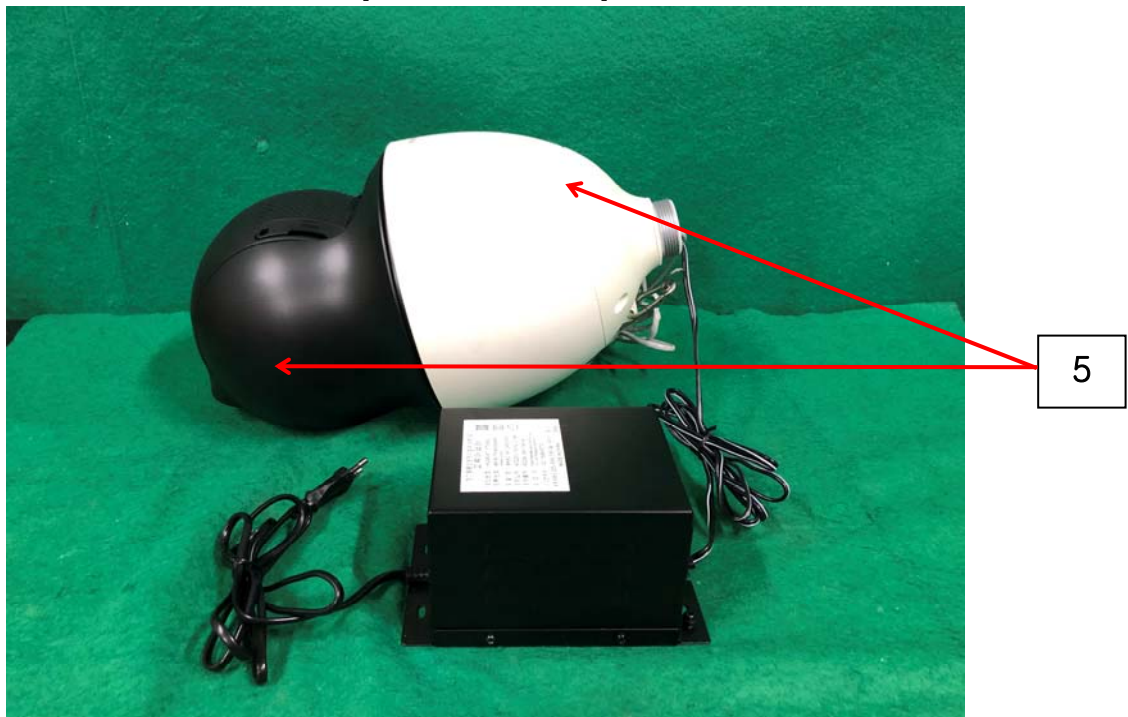
[시험기자재 우측면]
