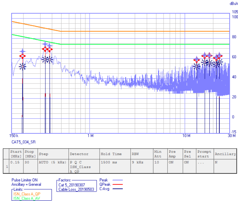
[POE_CAT. 5]
