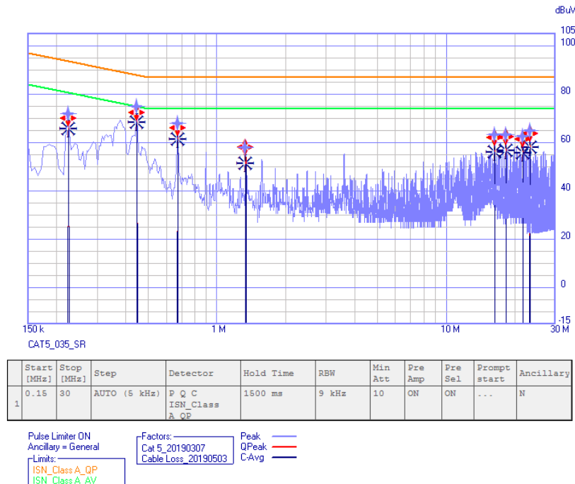
[POE_CAT. 5]
