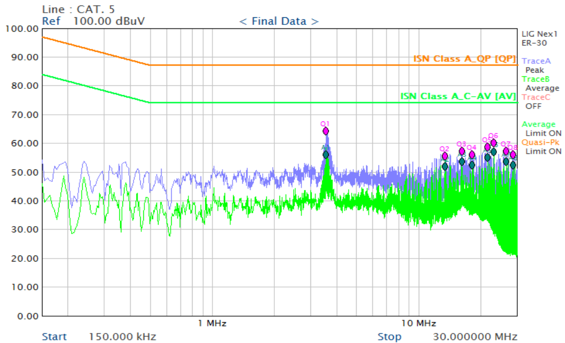
[POE_CAT. 5]
