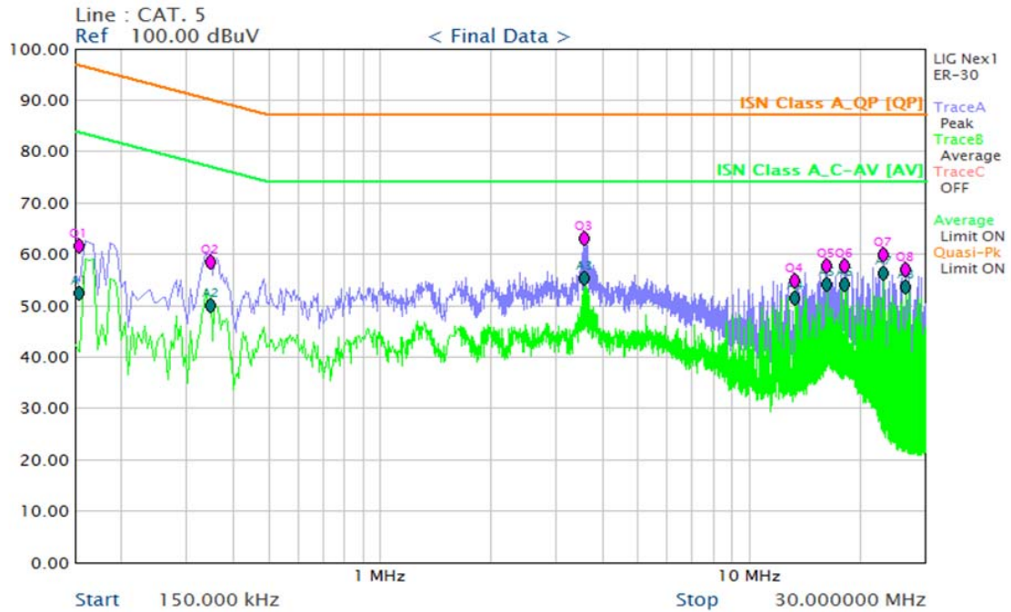
[DC IN_CAT. 5]
