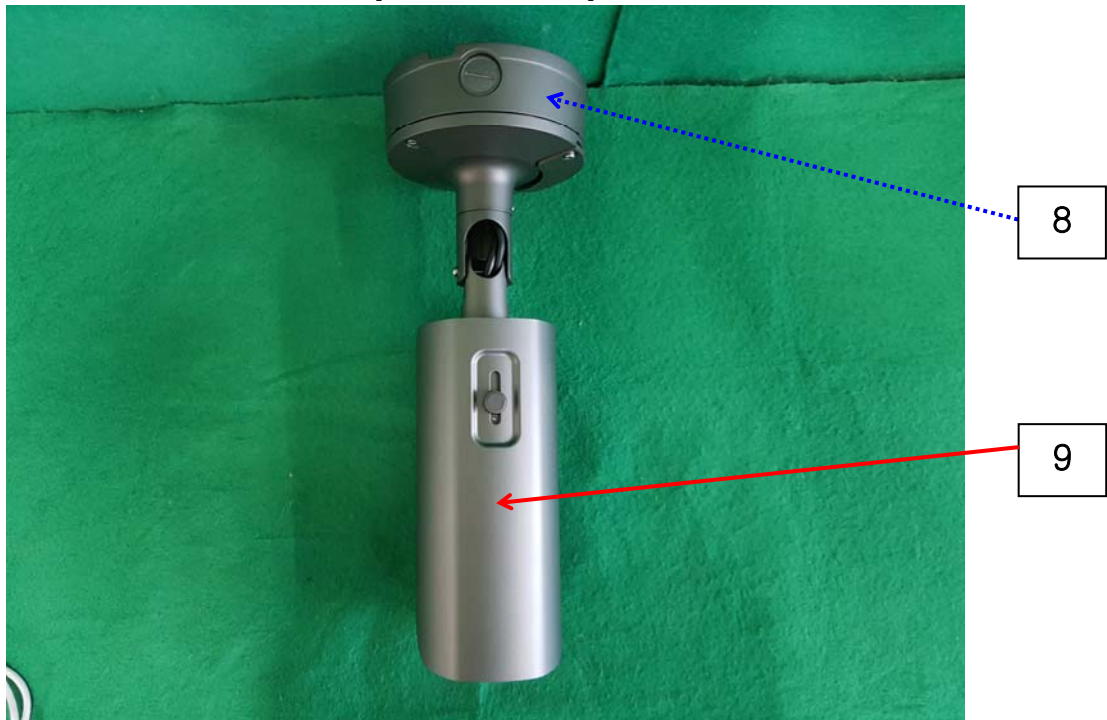
[시험기자재 윗면]
